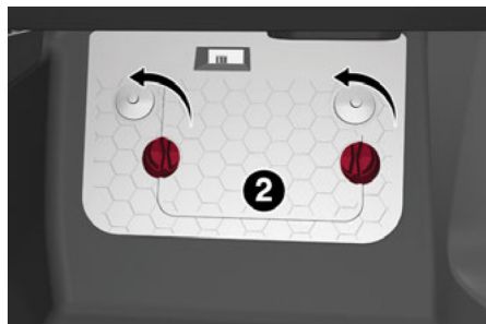
Enganches de fijación en el descansapiés
