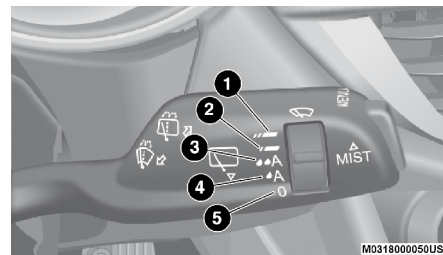
Interruptor de los limpiadores
