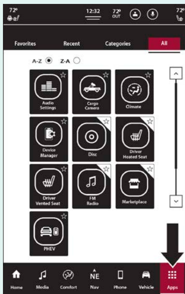
Modo aplicaciones Uconnect 5/5 NAV con pantalla de 12" (vertical)
