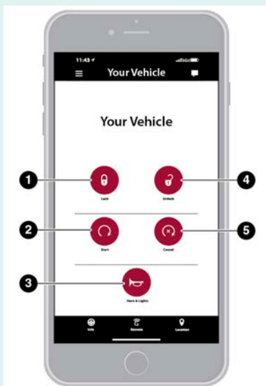
Comandos remotos
