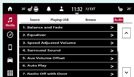
Ajustes de audio Uconnect 5 con pantalla de 7"
