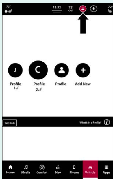
Menú Perfil 12"
