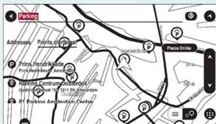
POI estacionamientos
