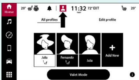
Menú Perfil 7"
