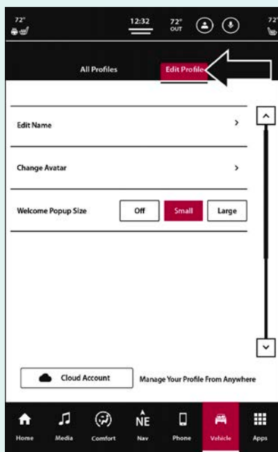
Editar perfil 12”
