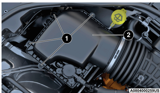
Conjunto de filtro de aire del motor
