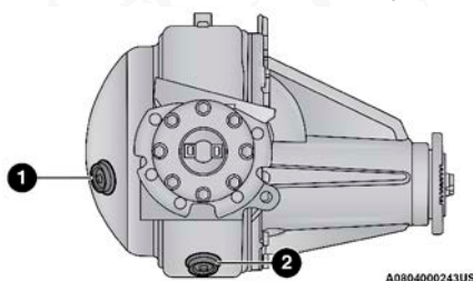
Orificios del eje trasero
