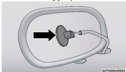
Retirando el portafoco de la lámpara
