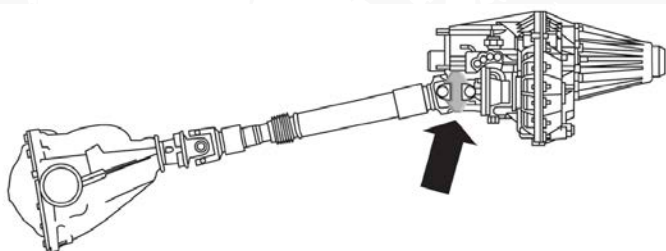
Lubricación de la flecha cardán frontal
