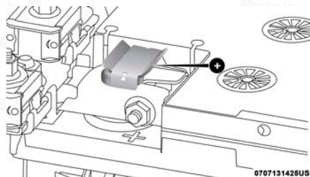
Ubicación de la terminal positiva (tipo 2)
