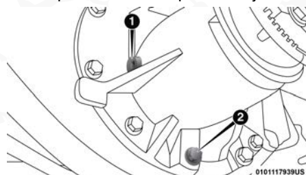
Orificios del eje trasero
