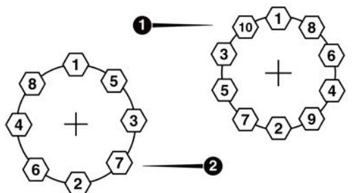
Patrón de apriete de 8/10 tuercas
