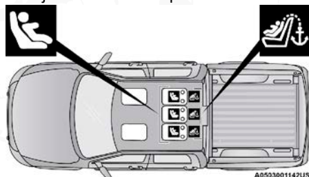
Posiciones LATCH en Crew Cab (doble cabina) banca dividida 60/40
