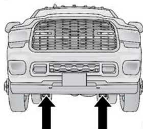
Colocación del gato en la parte delantera
