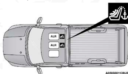
Ubicaciones de retractores de bloqueo automático en Cabina regular
