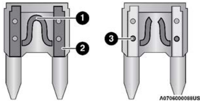
Fusibles de hoja
