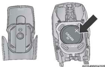
Ubicación de la batería del control
