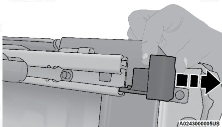
Retire la tapa al extremo del riel utilitario
