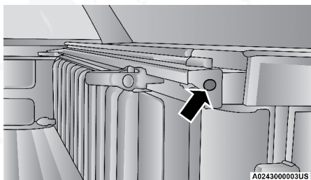
Ubicación del tornillo en la tapa al extremo del riel
