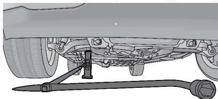
Punto de levantamiento delantero
