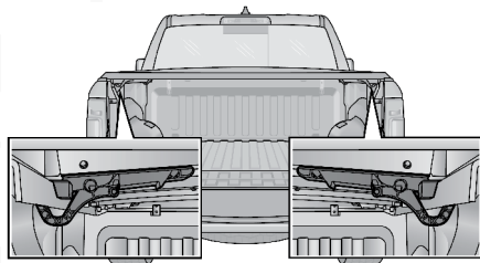
Deslice la palanca de bloqueo hacia adentro
