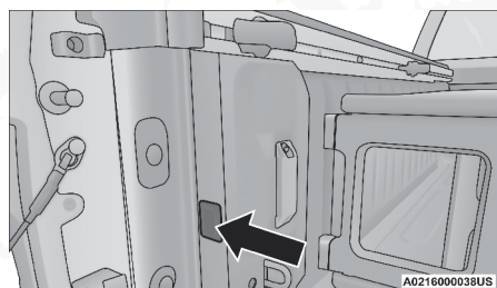
Interruptor de las luces dentro de la batea con RamBox
