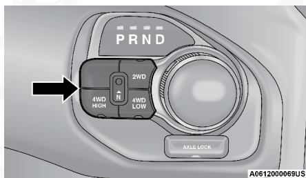
Interruptor de la caja de transferencia de 4 posiciones bajo demanda
