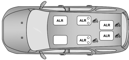
Segunda fila (asientos tipo capitán) (6 pasajeros) Ubicación retractor de bloqueo automático (ALR).
