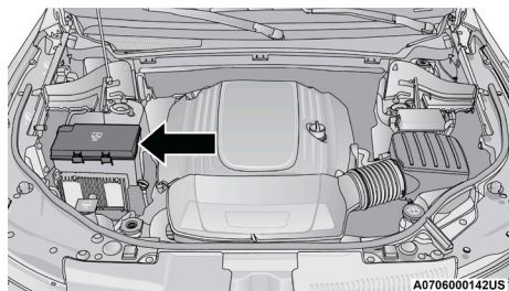
Ubicación del centro de distribución de potencia
