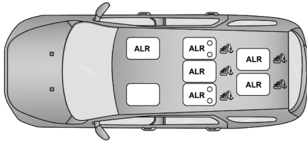
Segunda fila 60/40 (7 pasajeros) Ubicación retractor de bloqueo automático (ALR).
