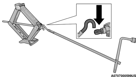
Ensamble del gato y la herramienta
