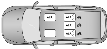
Segunda fila 60/40 (5 pasajeros) Ubicación retractor de bloqueo automático (ALR).
