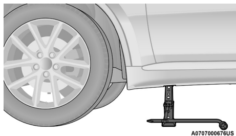
Punto de elevación delantero
