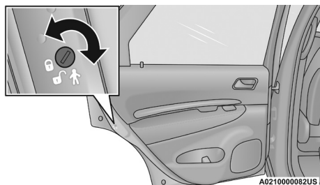
Función de protección para menores
