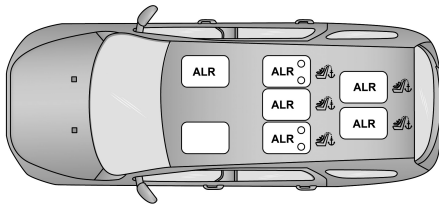
Segunda fila 60/40 (7 pasajeros) Ubicación retractor de bloqueo automático (ALR).
