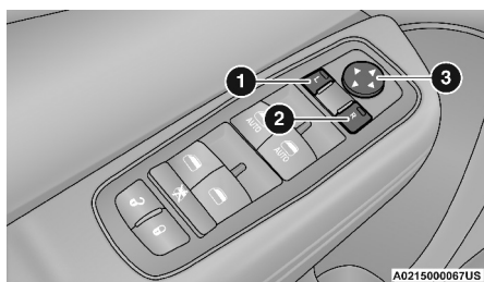
Interruptores de espejos eléctricos
