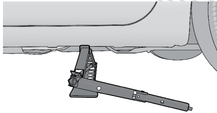
Punto de elevación trasero
