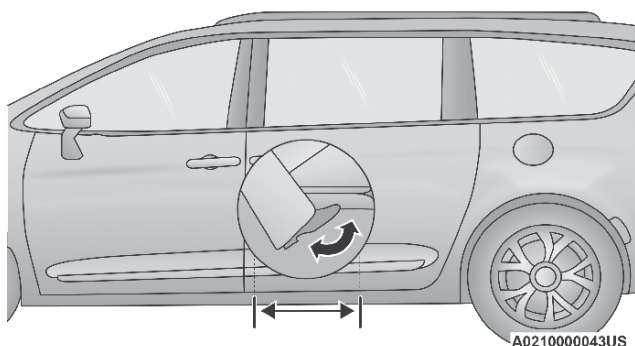
Característica de deslizamiento de puerta sin manos
