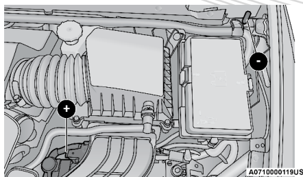
Ubicación de los polos de la batería
