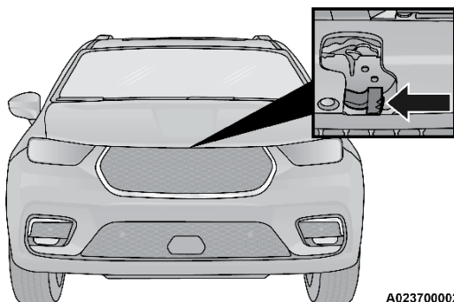
Ubicación del seguro del cofre
