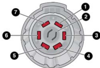
Conector de 7 clavijas
