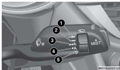
Interruptor de los limpiadores
