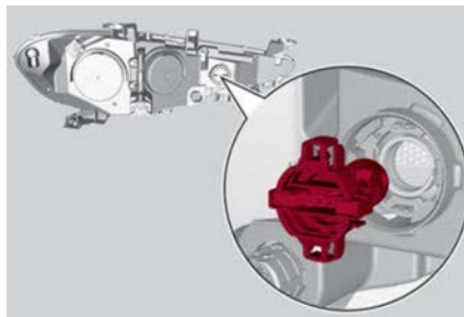
Ensamble del conector/foco
