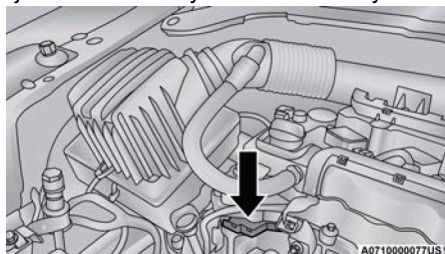
Tierra en el motor apropiada (Motor mostrado de forma ilustrativa)
