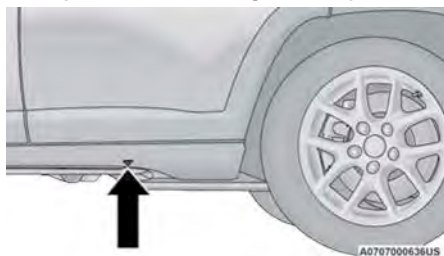
Punto de elevación en la parte trasera
