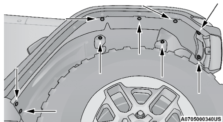
Cubierta interna de los arcos de rueda
