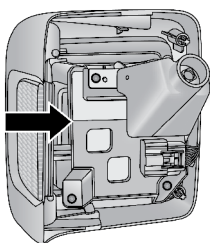
Ensamblaje del sujetador
