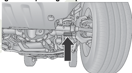
Punto de levantamiento con gato en la parte delantera
