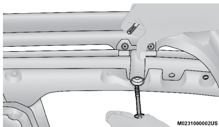
Retire los tornillos de la parte inferior del marco
