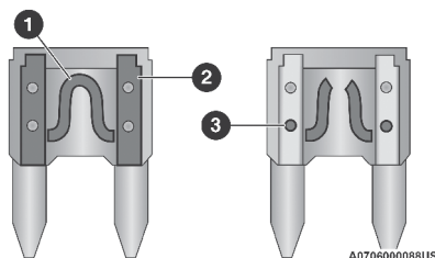
Fusibles de hoja
