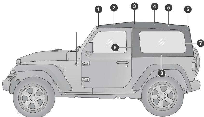
Vista lateral y componentes (versión de cuatro puertas)
