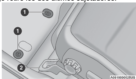
Piso y asiento delantero
