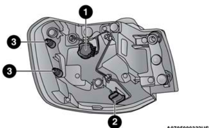
Parte trasera de la calavera
