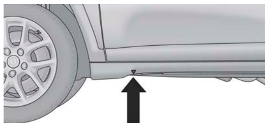
Dónde colocar el gato
