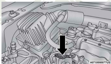
Punto de tierra en el motor apropiado
