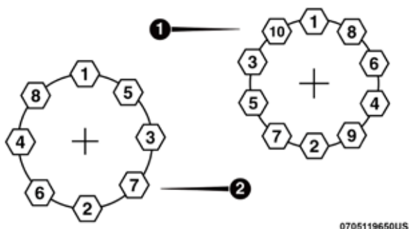
Patrón de apriete de 8/10 tuercas
