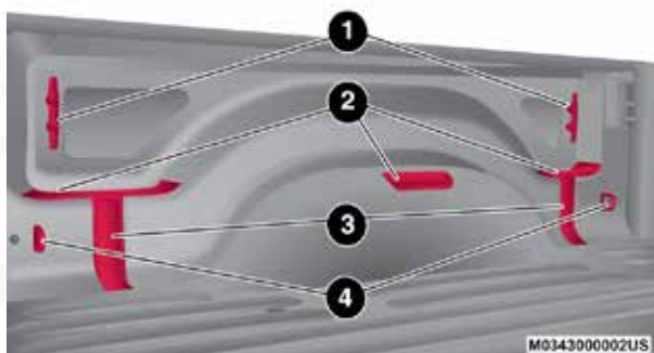
Características de la caja Pickup
