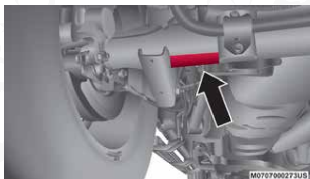
Punto de elevación en la parte trasera
