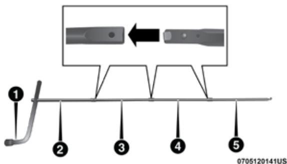
Ensamble para operar el gato
