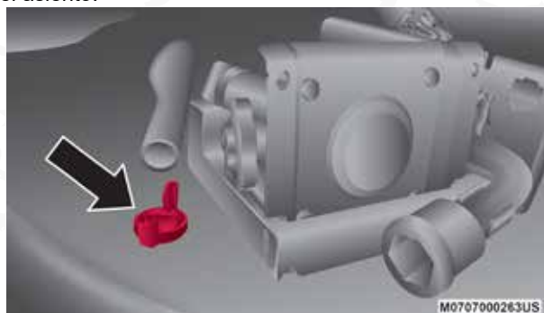
Perno de mariposa/Gato y herramientas
