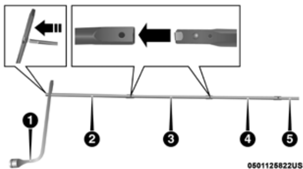
Ensamble para bajar/levantar la rueda de repuesto
