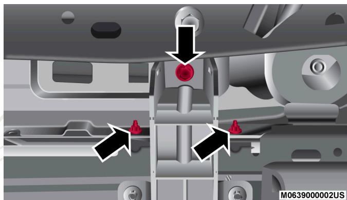
Tuercas laterales
