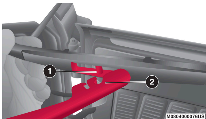
Hoja limpiadora retirada del brazo limpiador
