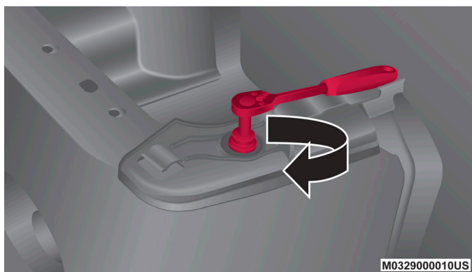
Instalación de los retenedores traseros
