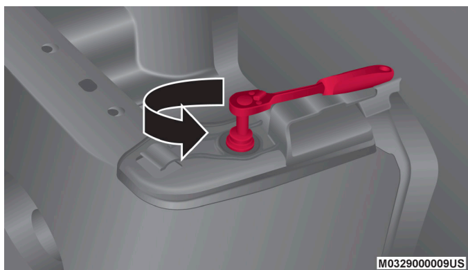
Retiro de los retenedores traseros
