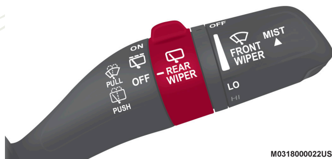
Control del limpiador/lavador trasero
