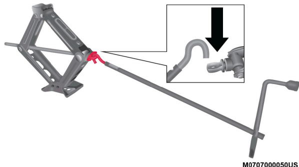
Gato ensamblado y herramientas
