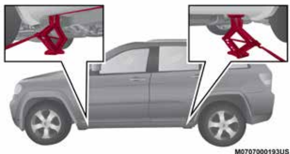
Puntos para colocar el gato
