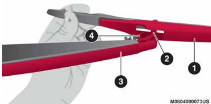
Pluma del limpiador retirada del brazo limpiador
