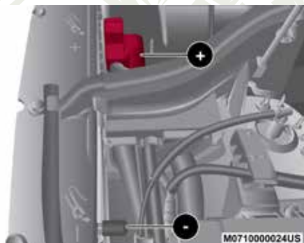
Postes remotos de la batería
