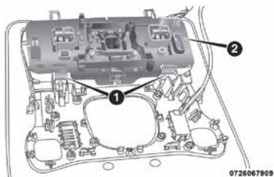
Compartimiento de las luces de cortesía frontales
