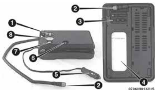
Componentes del kit de reparación
