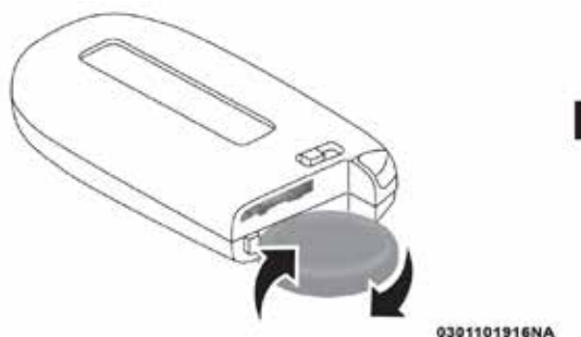
Separación de la cubierta usando una moneda
