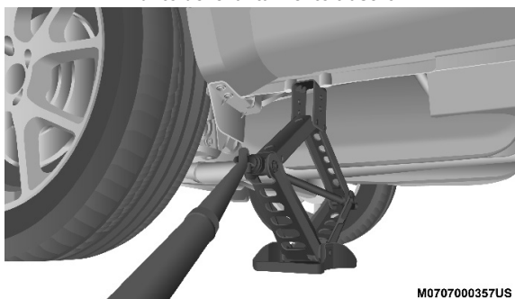
Colocación del gato parte trasera
