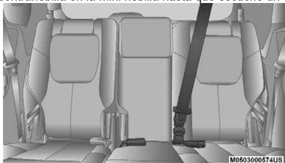
Conexión de la mini hebilla a la hebilla
