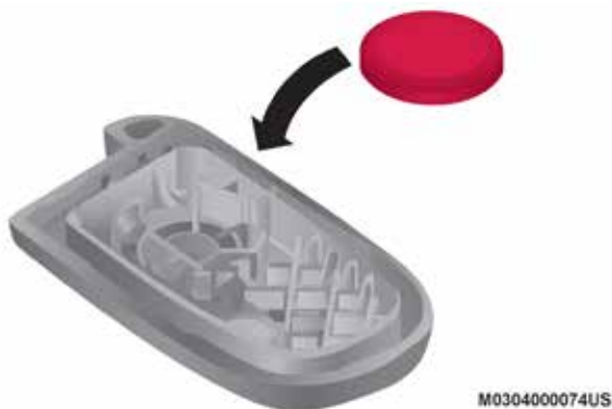
Separando la cubierta del transmisor con una moneda
