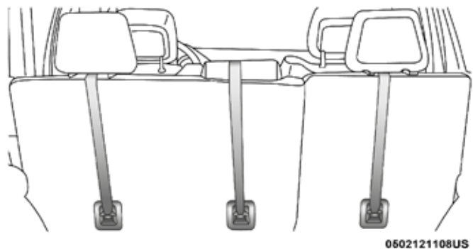
Montaje de los anclajes de correa superior (5 pasajeros)
