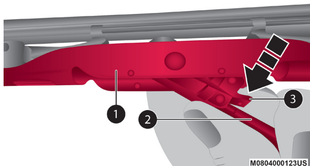
Hoja del limpiador con la pestaña de liberación en posición de desbloqueo
