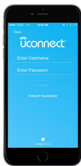
App móvil
