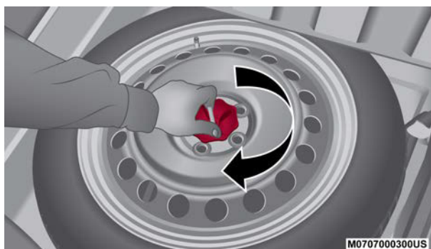
Apriete del sujetador de la llanta
