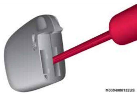
Separación de la cubierta con un desarmador de punta plana
