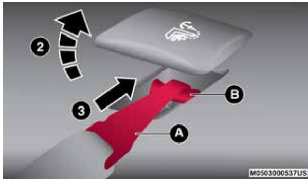
Montaje de la correa de sujeción
