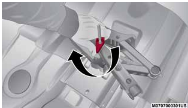
Apriete del sujetador del gato
