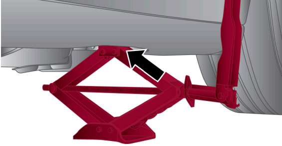
Localización para levantamiento con gato delantera
