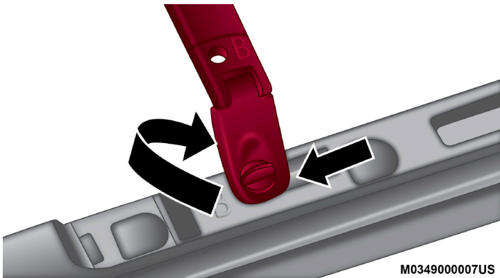
Instalación de las barras
