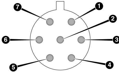
Conector de siete vías
