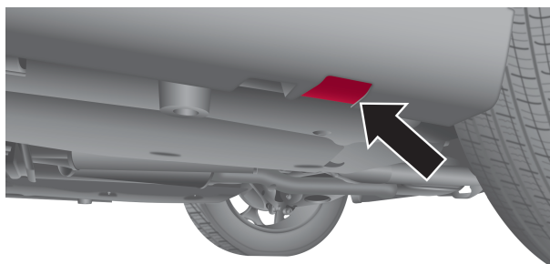
Colocación del gato en la parte frontal
