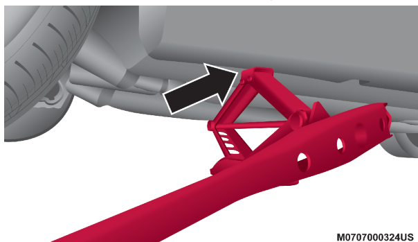
Colocación del gato en la parte frontal
