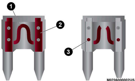
Hoja del fusible
