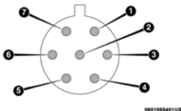
Conector de 7 clavijas
