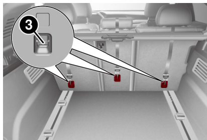
Ubicación de anclajes para correa superior
