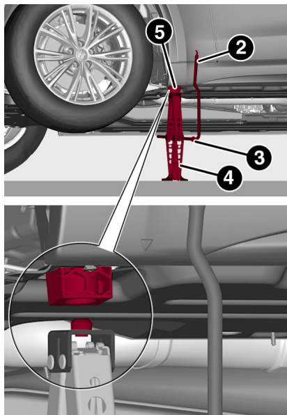
Posición del gato
