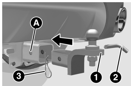
Ranura y receptor del remolque
