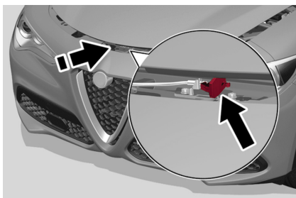
Seguro de liberación del cofre
