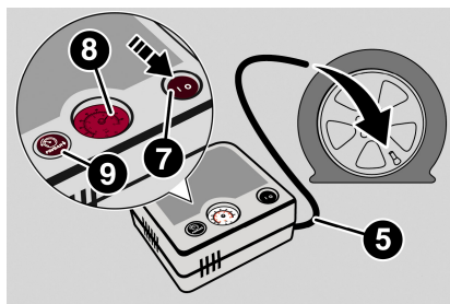
Componentes del compresor
