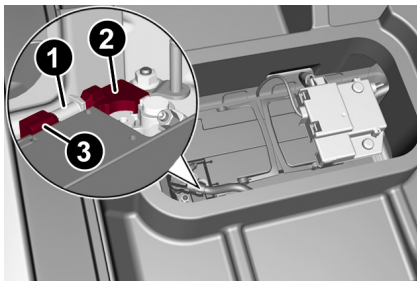
Suministro de energía a la batería
