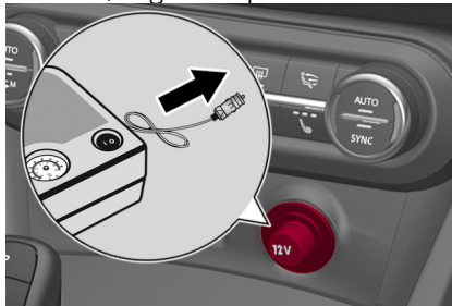
Conectando el compresor
