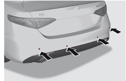
Ubicación de los sensores traseros
