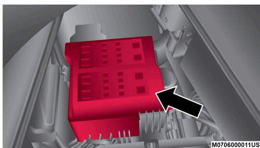
Cubierta de la cavidad trasera de los fusibles del área de carga
